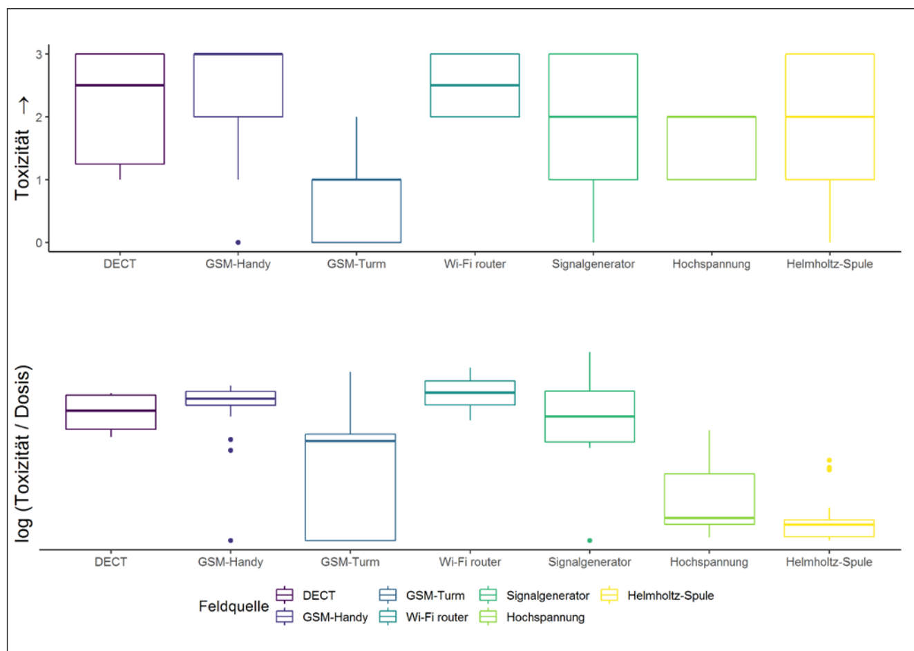
Abb. 11: Oben: Mutmaßliche Toxizität für Insekten nach EMF-Typ (Schätzwert). Untere Grafik: Relative Schädlichkeit nach EMF-Typ (Schätzwert), normalisiert auf die Strahlungsdosis, d.h. geteilt durch Produkt aus Feldstärke mit Expositionsdauer [V/m × min], auf einer log 2 -Skala dargestellt. Zum Vergleich der HF-EMF mit den LF-EMF wurden alle Werte der magnetischen Feldstärke [T] in elektrische Feldstärke [V/m] konvertiert (siehe Anhang).
