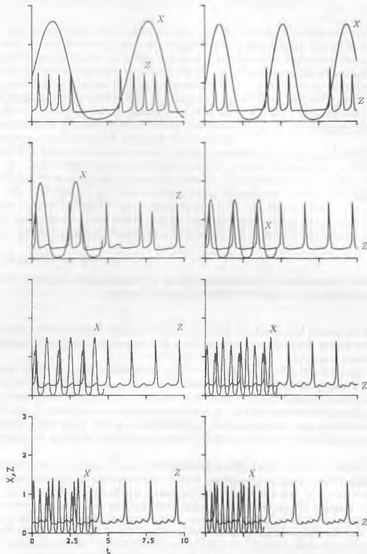
Bild 3: Oszillationsdiagramme der Variablen X, Z , v. l. o. r. u.: \frac{5}{1}, \frac{3}{1}, \frac{3}{2}, \frac{1}{1}, \frac{1}{2}, \frac{1}{3}, \frac{1}{4}, \frac{1}{5} -Resonanzen.
